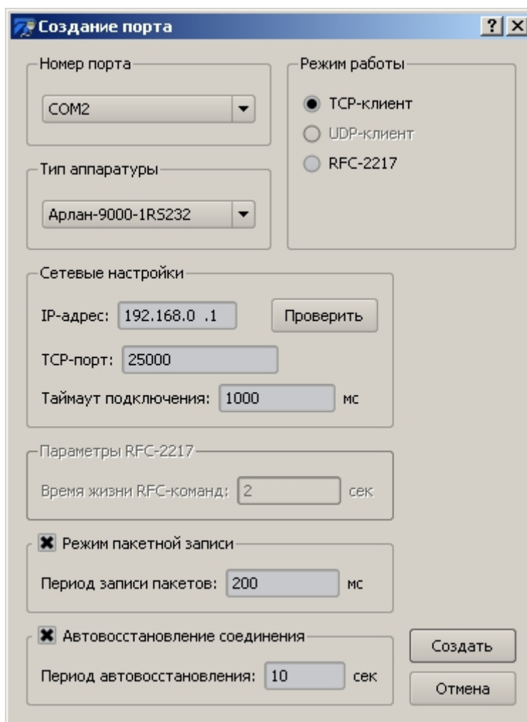
Рисунок 2 - Окно добавления виртуального СОМ-порта
